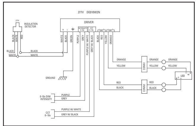
277V DE010W2N
