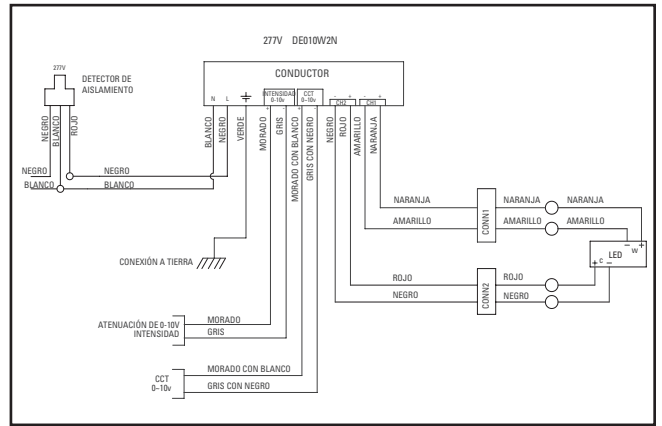
277V DE010W2N
