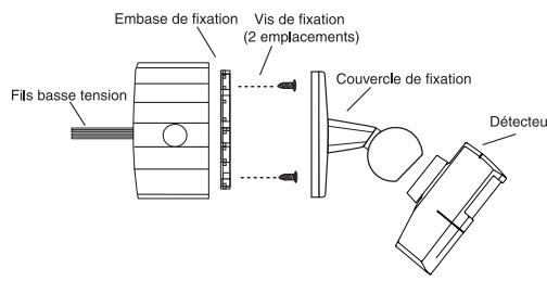
Détecteur de présence fixé sur boîte octogonale
