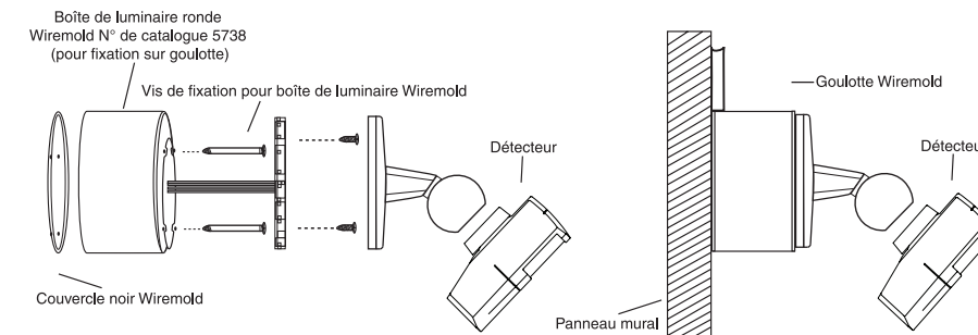
Détecteur de présence fixé sur boîte de luminaire ronde avec goulotte
