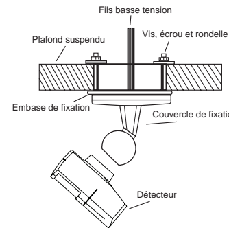
Détecteur de présence fixé sur plafond suspendu
