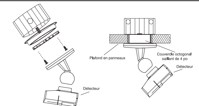
Détecteur de présence fixé sur boîte octogonale avec virole pour enduit
