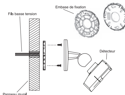
Détecteur de présence fixé sur panneau mural
