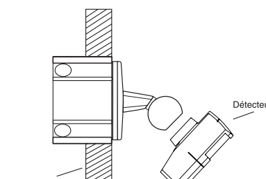
Détecteur de présence fixé sur plafond suspendu
