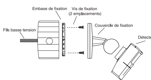
Détecteur de présence fixé sur boîte octogonale
