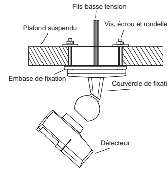
Détecteur de présence fixé sur plafond suspendu
