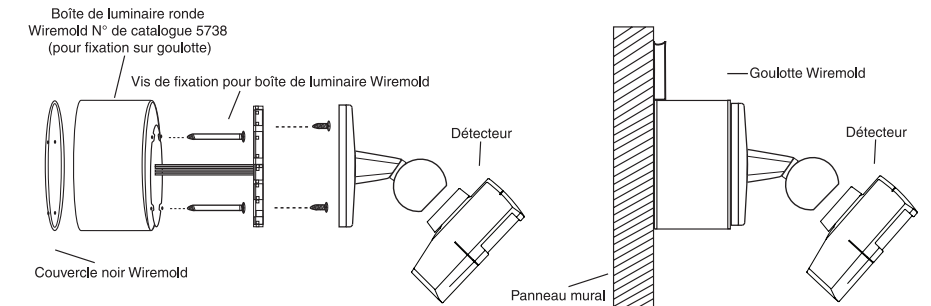
Détecteur de présence fixé sur boîte de luminaire ronde avec goulotte
