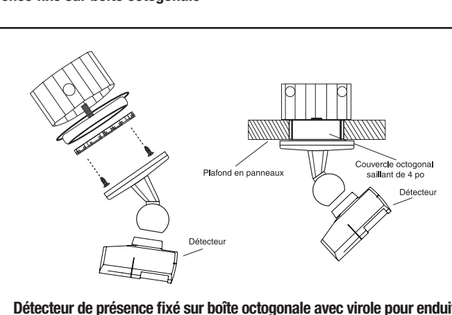
Détecteur de présence fixé sur boîte octogonale
