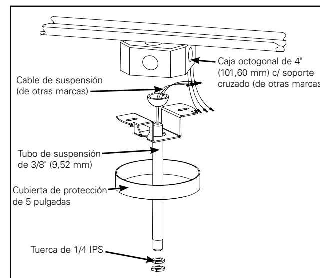
Figura 1. Alimentación
