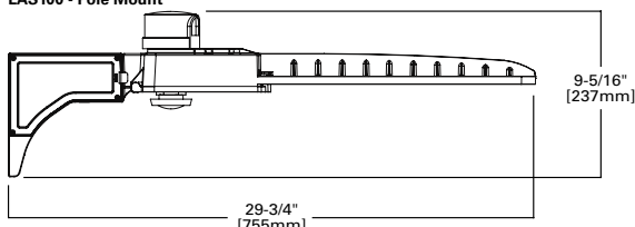
LAS100 - Pole Mount
