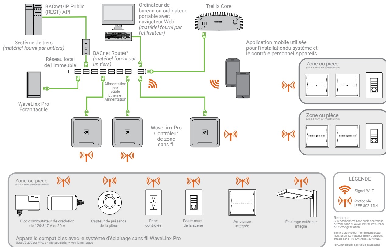
Figure 2. Installation en entreprise
