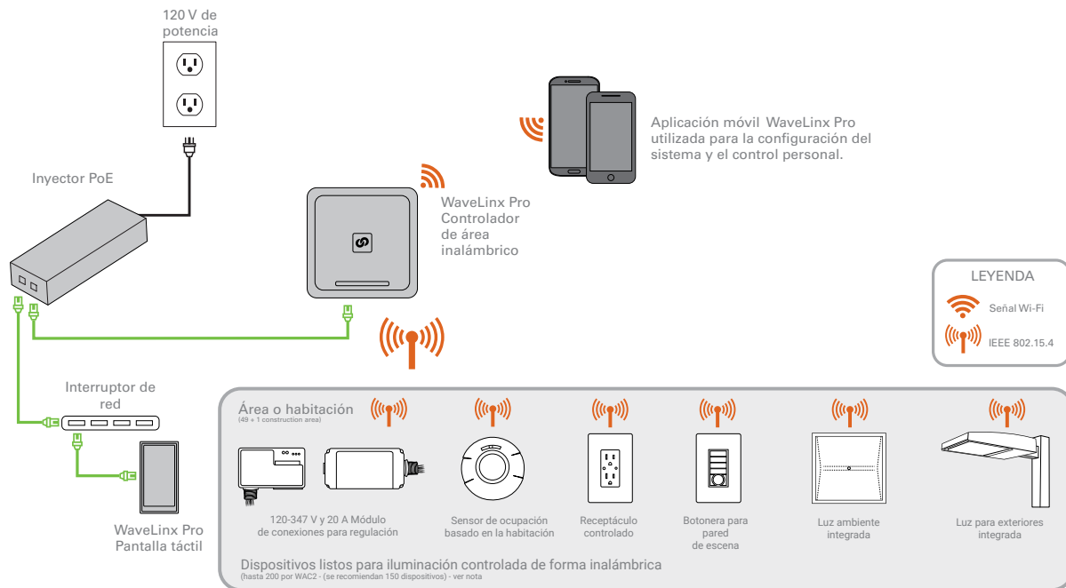
Figura 1 Instalación independiente del WAC
