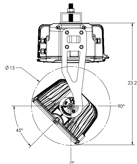
4a Pendant Mount
